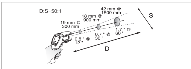
Рисунок 5. Расстояние и размер измеряемой области
