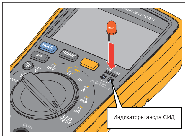
Рисунок 4. Гнезда проверки светодиодов
